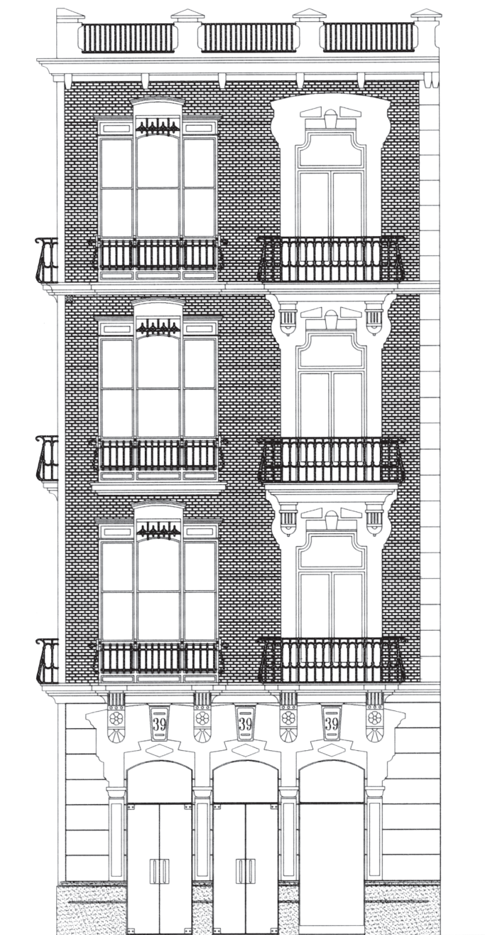
Alzado reformado frontal Edificio Alessón calle Jara. JAG.
